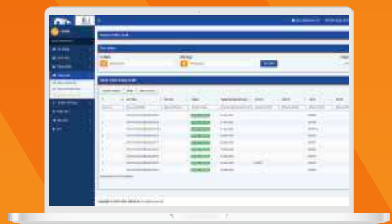
FMS
